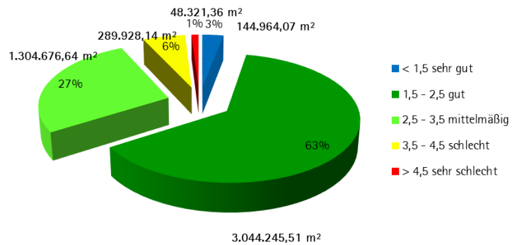
Zustandsverteilung im Nebennetz 2009 - Gesamtwert
